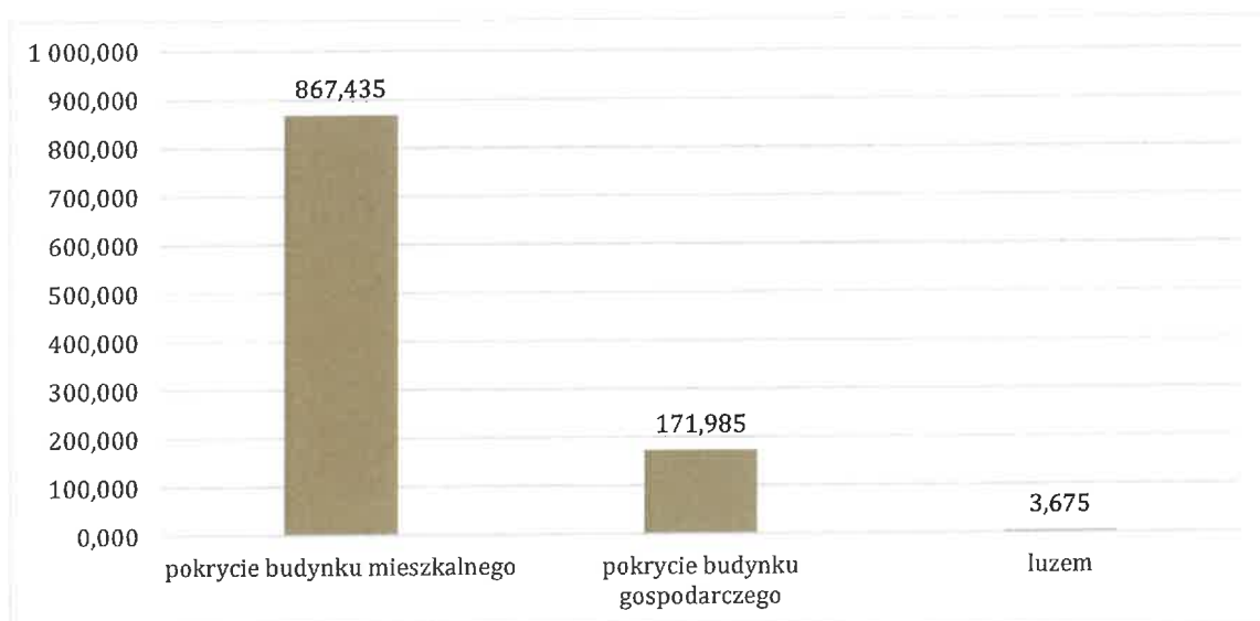
Rysunek 9 Ilość wagowa wyrobów zawierających azbest z podziałem na pokrytą powierzchnię na budynkach mieszkalnych, gospodarczych i innych na terenie gminy Wilkowice [Mg]
